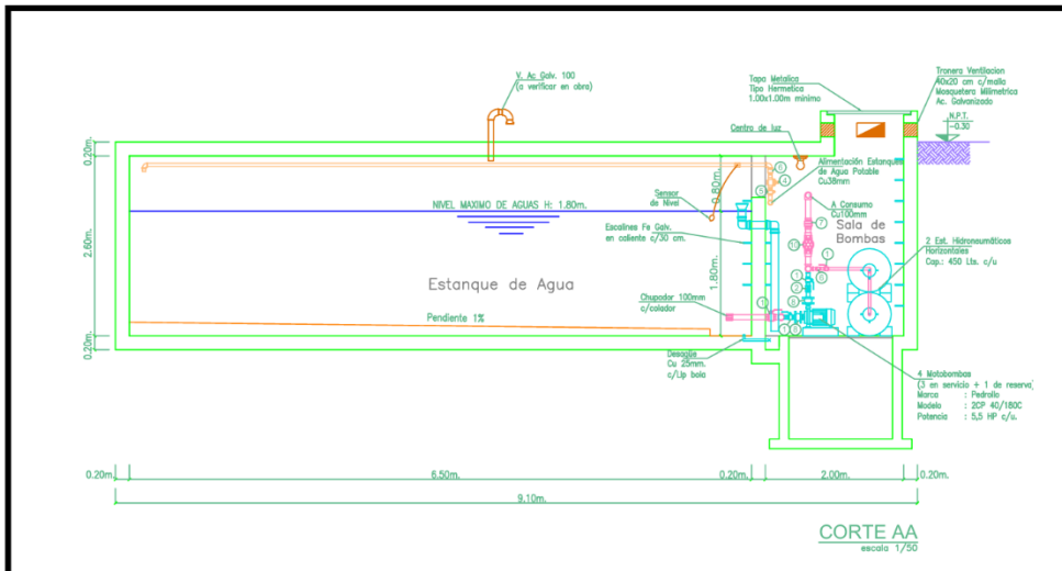
IMAGEN 06: Detalle de los estanques, vista en corte.
