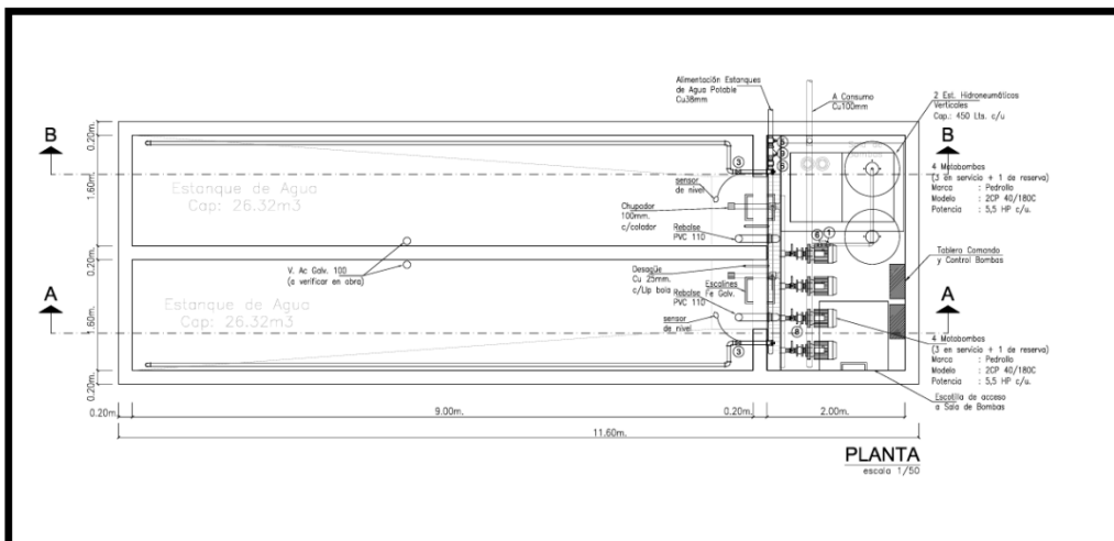
IMAGEN 07: Detalle de los estanques, vista de planta.
